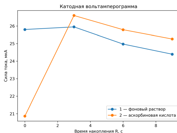
Рисунок 1 — Катодная вольтамперограмма аскорбиновой кислоты ( 1 \times 10^{-3} М) в 0,1 М фосфатном буфере (pH 6,8); скорость развертки 50 мВ/с; ртутно-плёночный электрод
