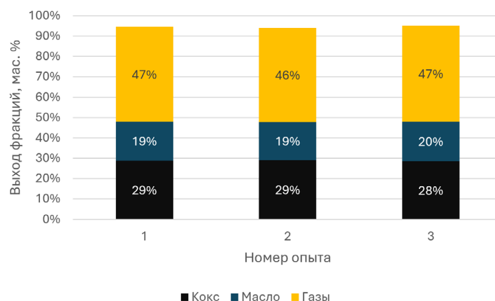
Рисунок 3 – Массовый баланс пиролиза
