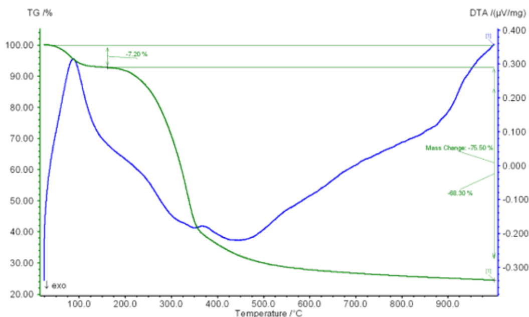
Рисунок 2 – ТГА-анализ лузги подсолнечника
