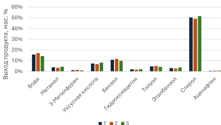
Рисунок 5 – Результаты анализа GC-MS пиролизного масла
