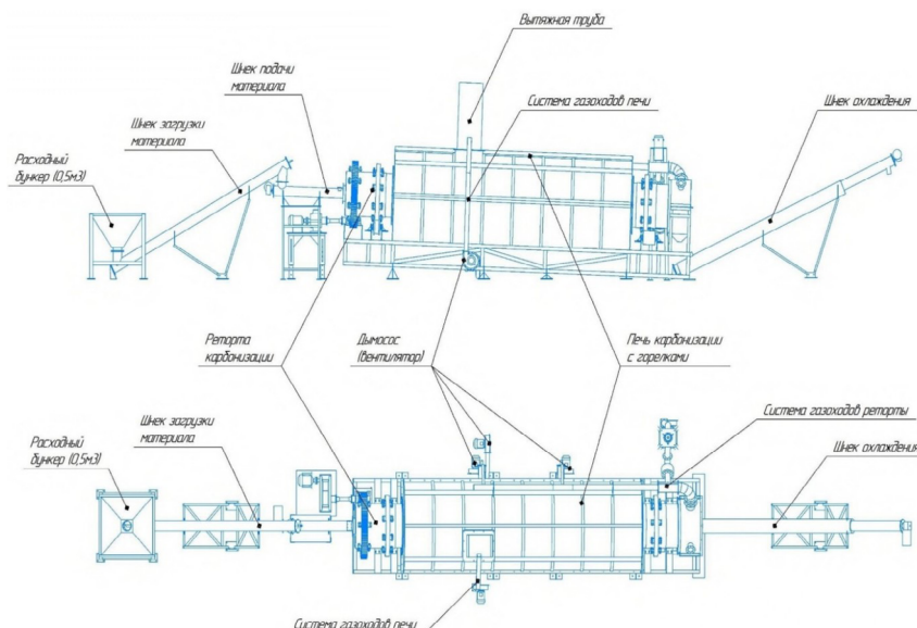
Рисунок 9 – Принципиальная схема комплекса карбонизации лузги подсолнечника «МОДУЛЬ КАРБОНИЗАЦИИ БИОМАССЫ. Тип СП - К400»
