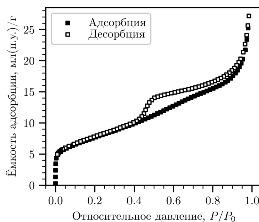
Рисунок 6 – Изотерма адсорбции–десорбции азота при 77 К карбонизатом лузги подсолнечника
