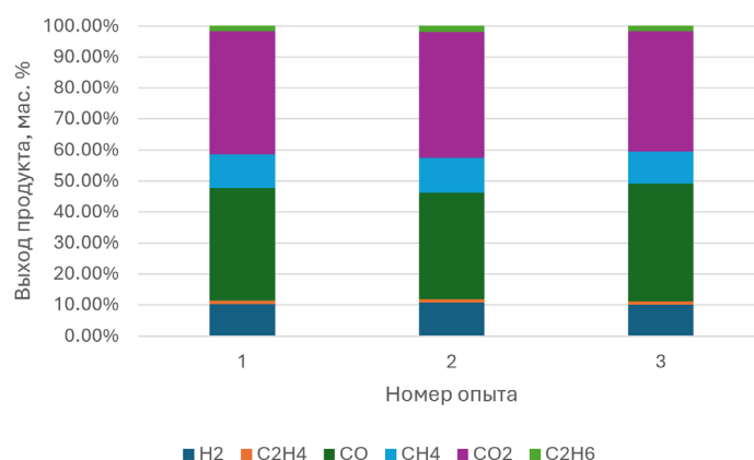
Рисунок 4 – Состав газовой фракции пиролиза
