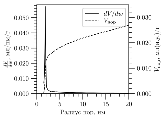
Рисунок 7 – Кривые распределения пор по размерам и суммарного объёма пор, рассчитанные методом ВН для карбонизата лузги подсолнечника
