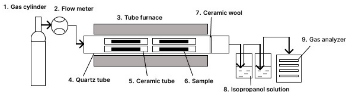
Рисунок 1 – Схема пиролиза лузги подсолнечника в трубчатой печи с неподвижным слоем
